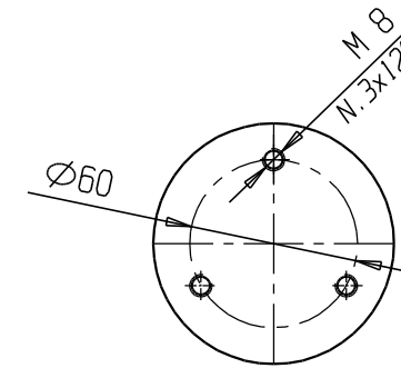
VISTA DA A VIEW A
